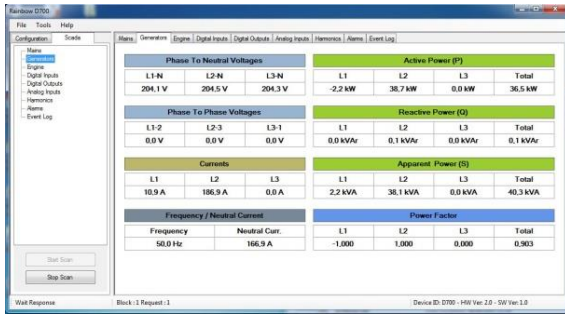
Écran Scada
